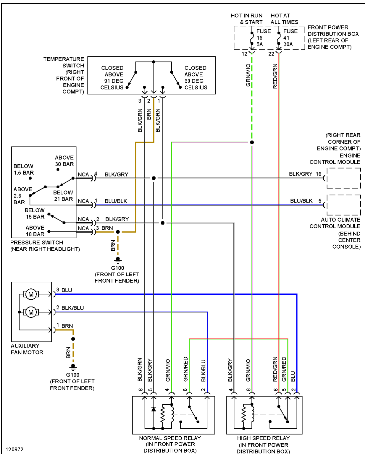
Fig. 18: Cooling Fan Circuit
